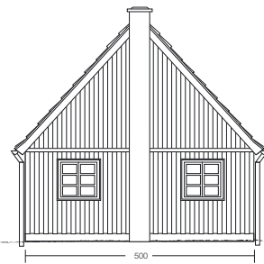
1:50 GAVL MOD ØST
